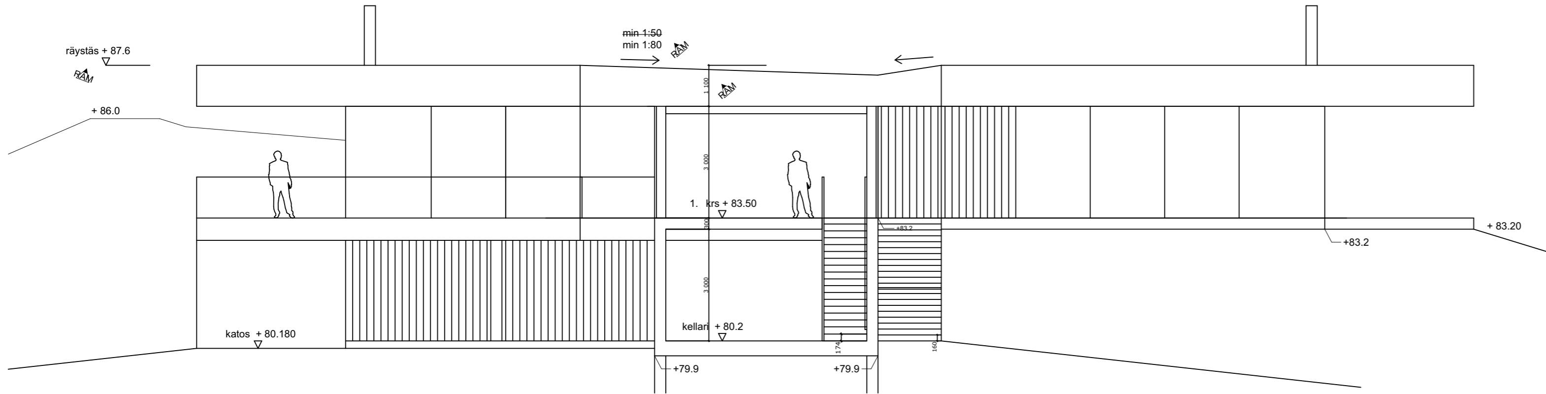
Leikkaus A-A
